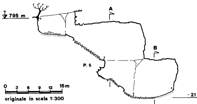
SEZIONE LONGITUDINALE
